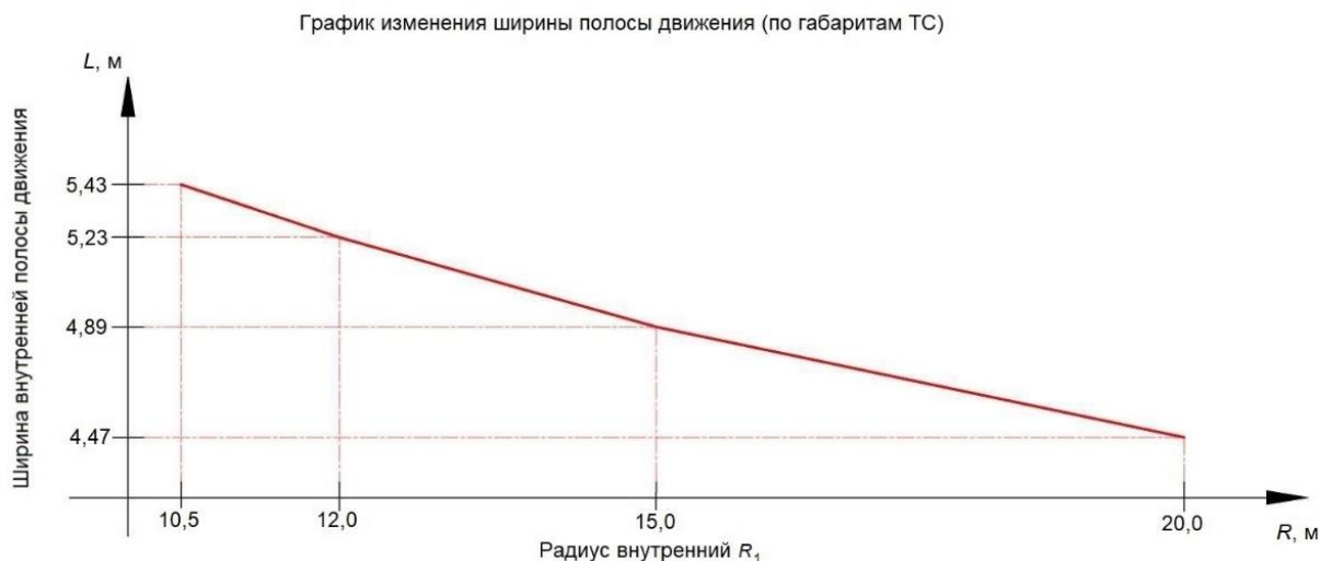
Рисунок 7 – Зависимость ширины полосы движения от радиуса для расчетного автомобиля A16
