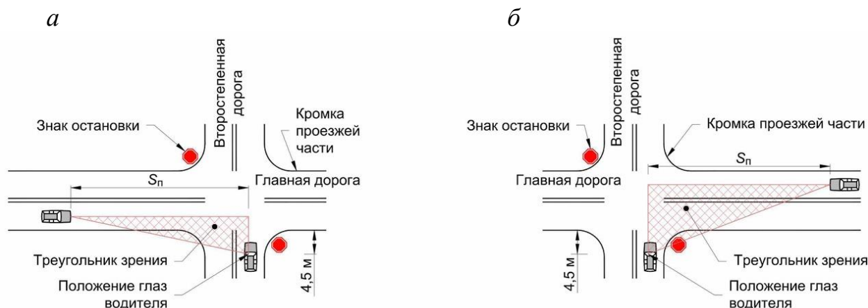
а – треугольник видимости при приближении автомобиля по главной улице или дороге справа; б – треугольник видимости при приближении автомобиля по главной улице или дороге слева
