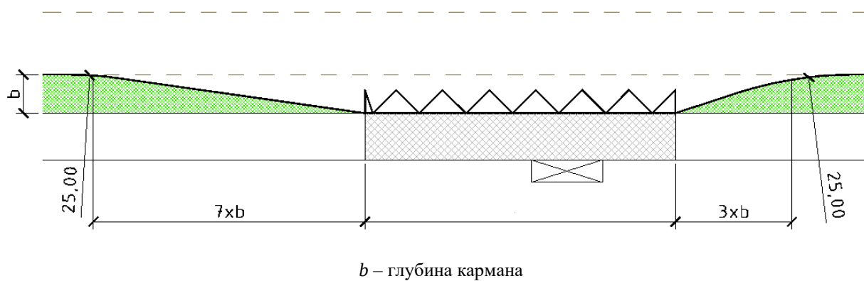
Рисунок В.1 – Остановочный пункт с параллельным карманом
