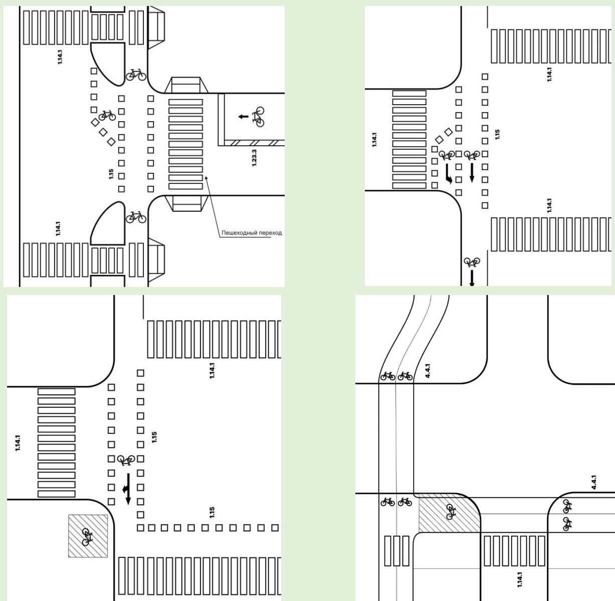
Рисунок 8 – Схема размещения площадок для ожидания разрешающего сигнала светофора
