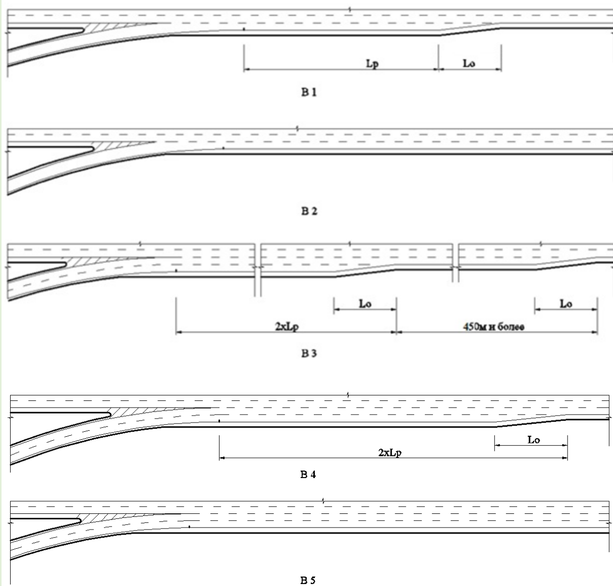
Рисунок Б.6 – Схемы участков слияния транспортных потоков
