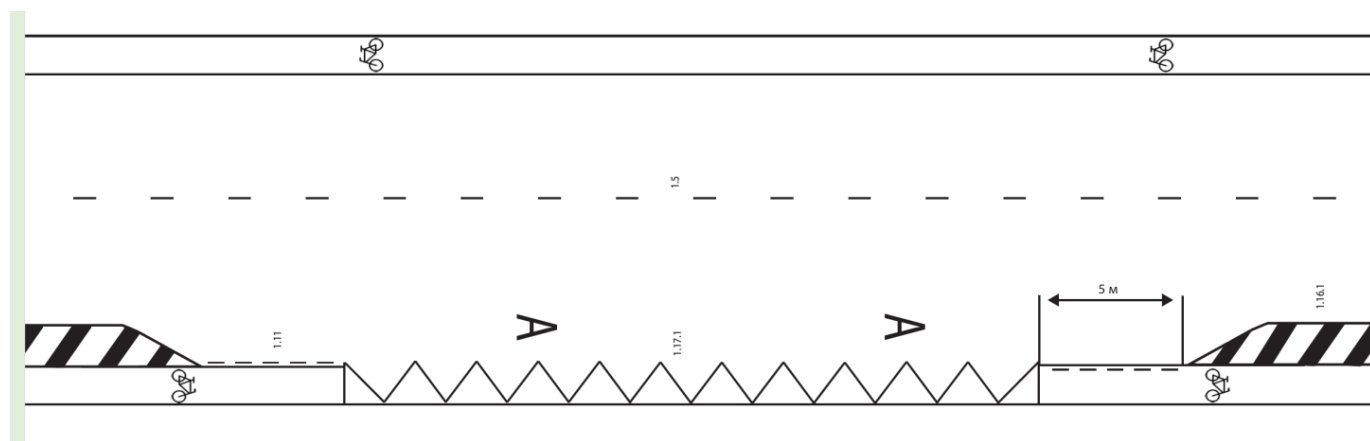
Рисунок 10 – Схема прерывания велосипедной полосы или велосипедной дорожки в зоне посадочной площадки
