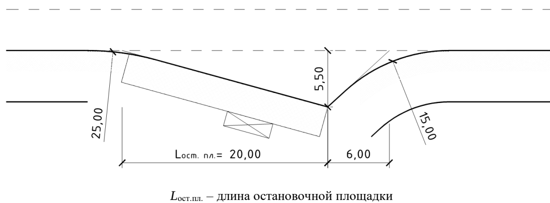
Рисунок В.2 – заездной пункт с карманом под углом к проезжей части
