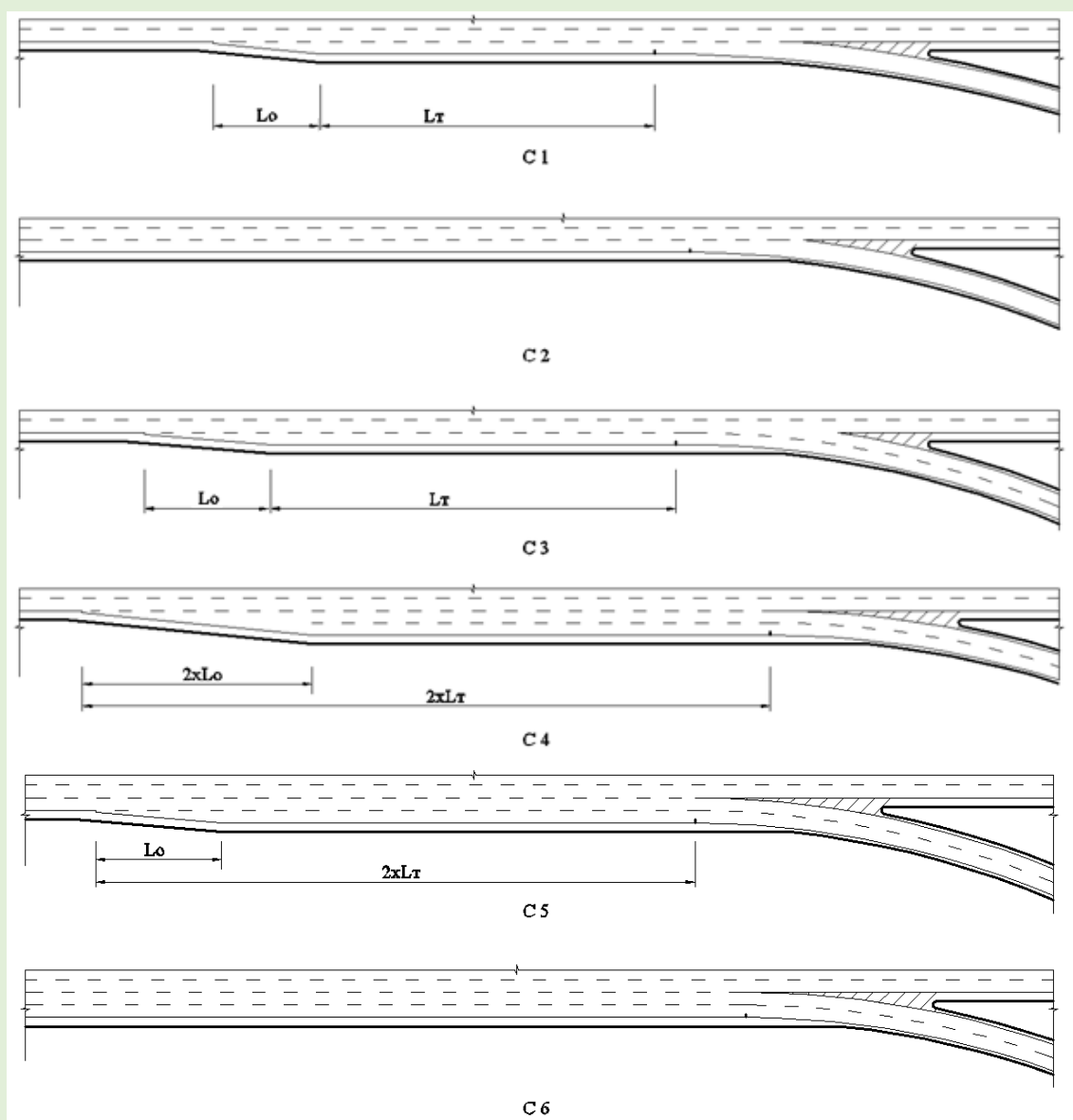
Рисунок Б.1 – Схемы участков разделения транспортных потоков
