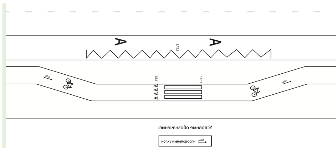
Рисунок 9 – Схема размещения велокоммуникаций в обход посадочной площадки
