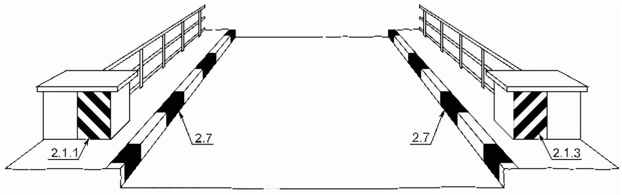
Рисунок В.23 - Пример нанесения разметки 2.1.1, 2.1.3 и 2.7
