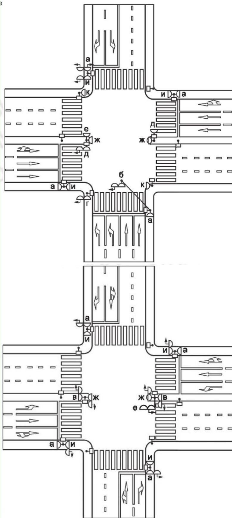
а-к - места установки светофоров по 7.4.1 Рисунок В.26 - Места установки светофоров
