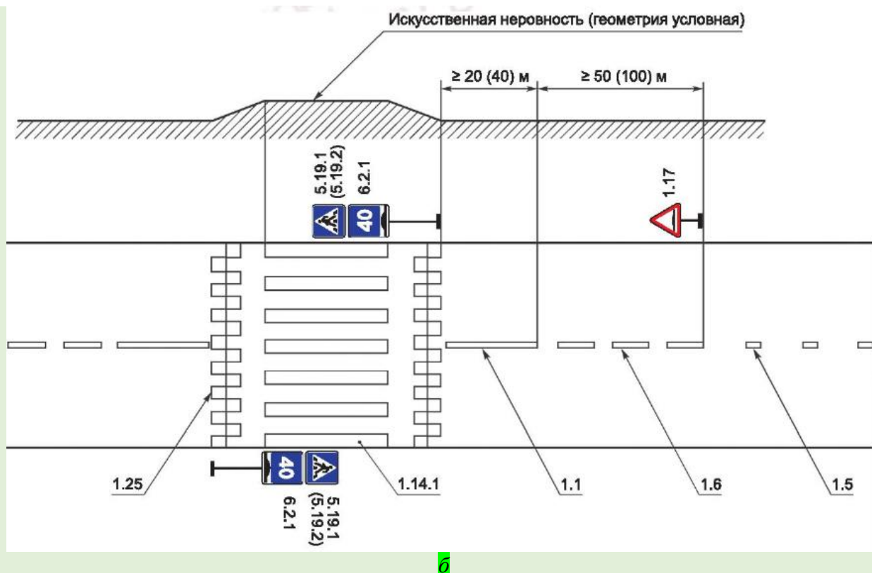
Рисунок В.21 – Примеры нанесения разметки 1.25
