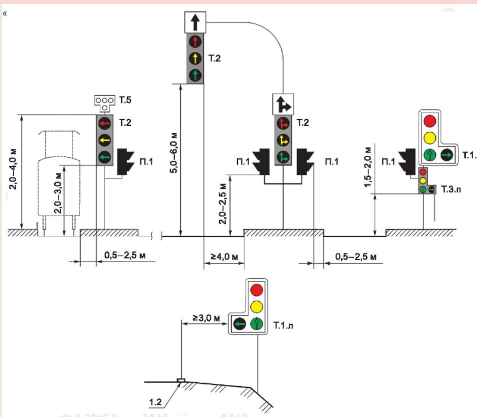
Рисунок В.25 - Примеры установки светофоров различных типов и исполнений
