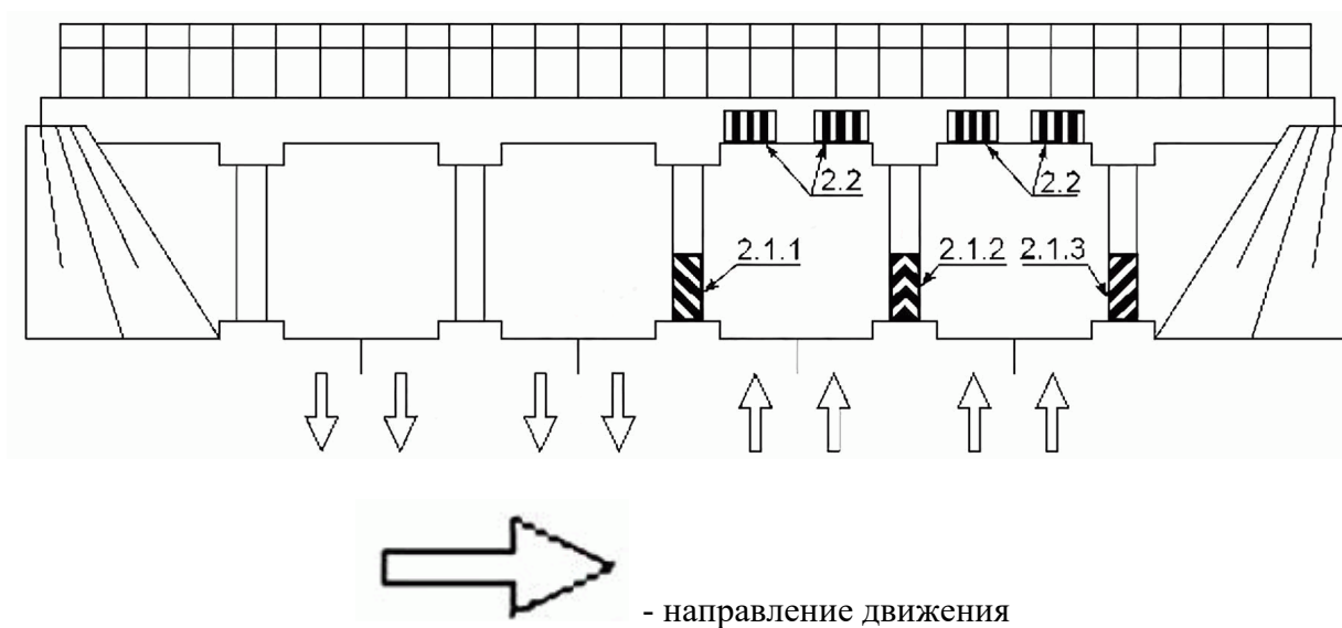
Рисунок В.22 - Пример нанесения разметки 2.1 и 2.2
