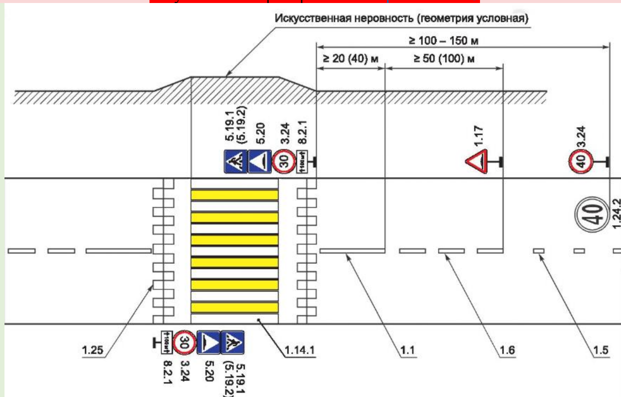
Рисунок В.21 - Пример нанесения разметки 1.25
