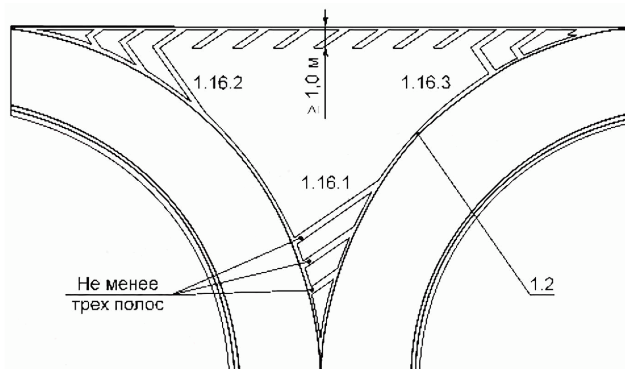
Рисунок В.12 - Пример нанесения разметки 1.16.1-1.16.3
