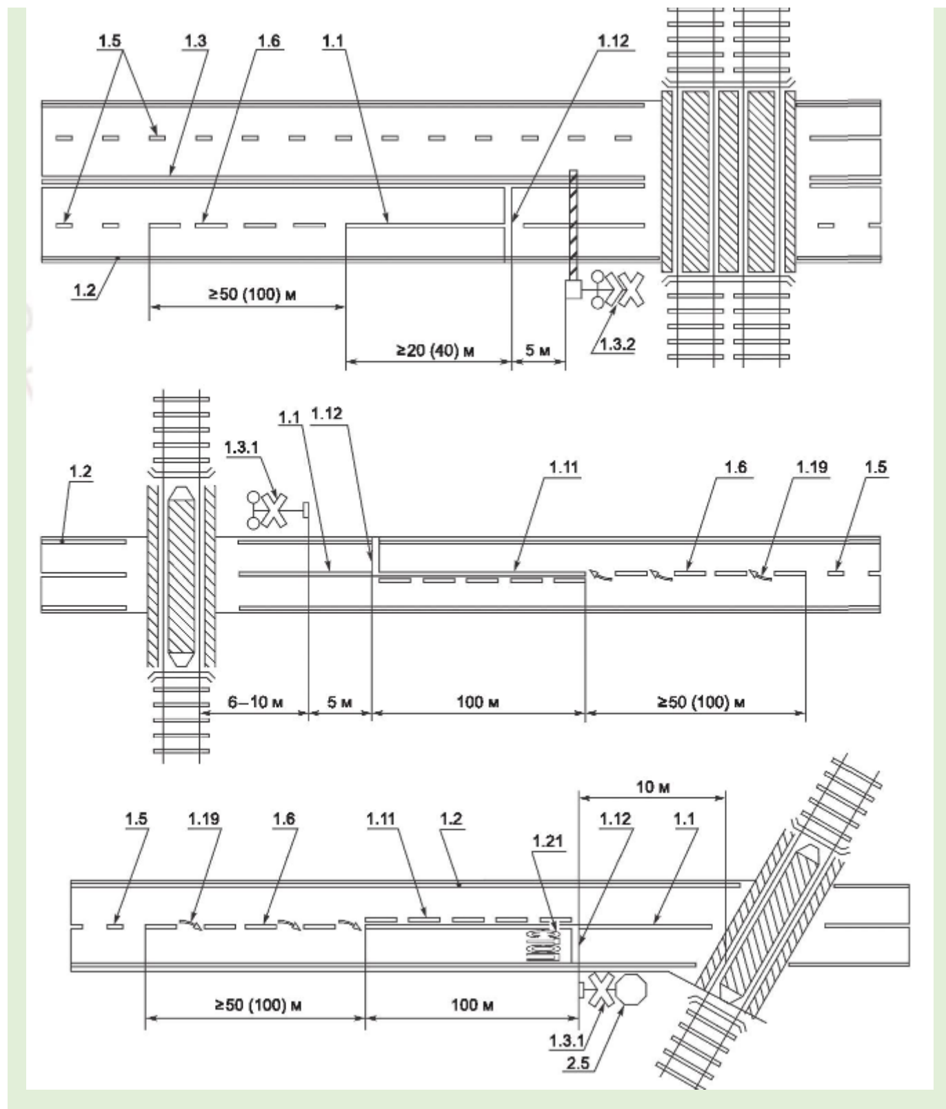
Рисунок В.18 - Примеры разметки участка дороги на подъезде к железнодорожному проезду
