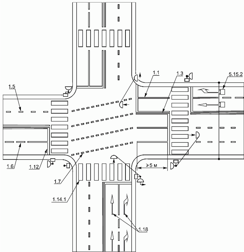
Рисунок В.9 - Пример нанесения разметки на регулируемом перекрестке
