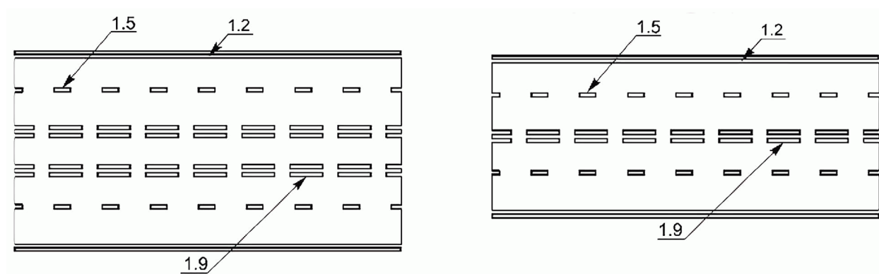
Рисунок В.17 - Примеры нанесения разметки 1.9
