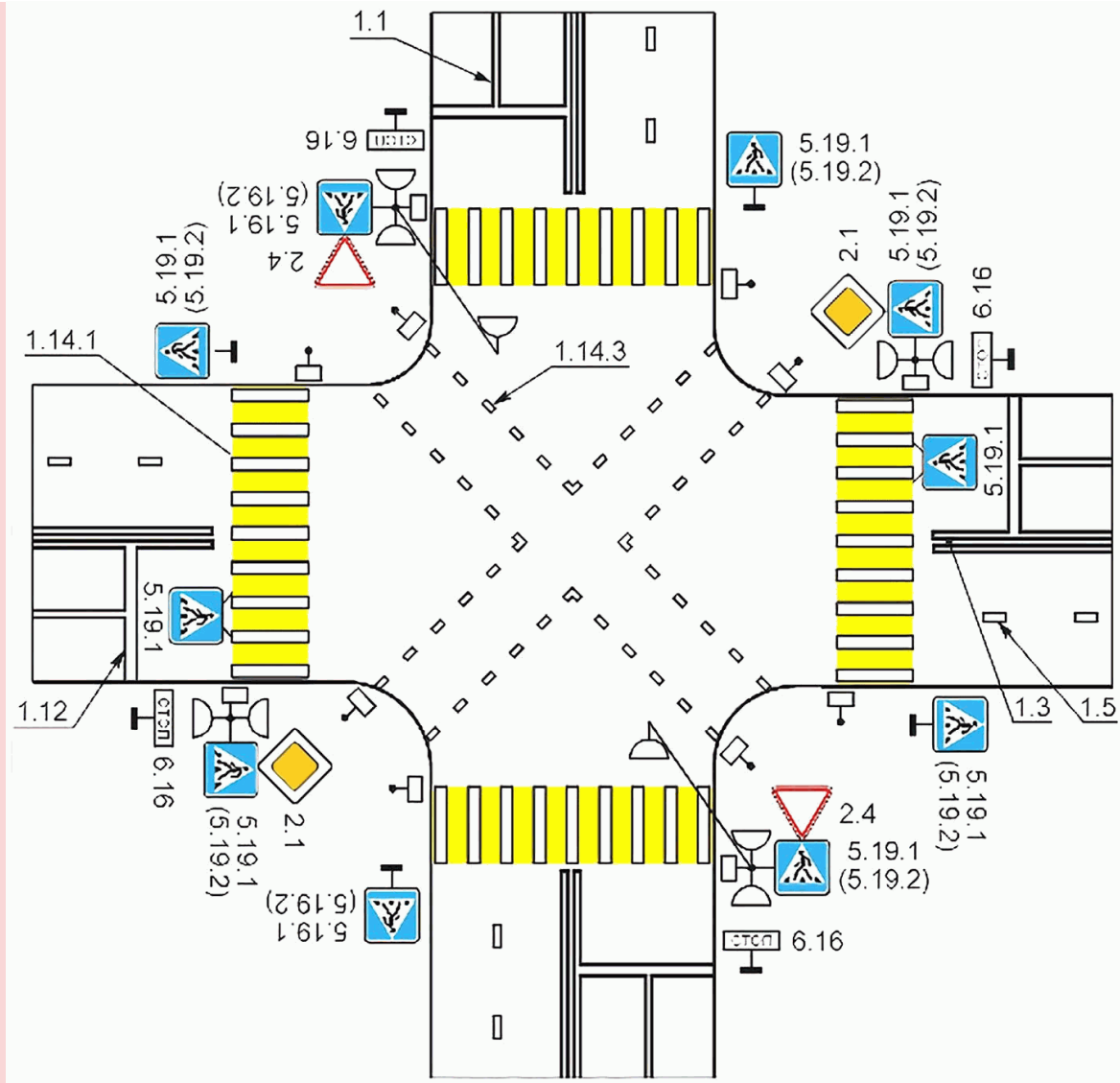
Рисунок В.19 - Пример нанесения диагонального пешеходного перехода
